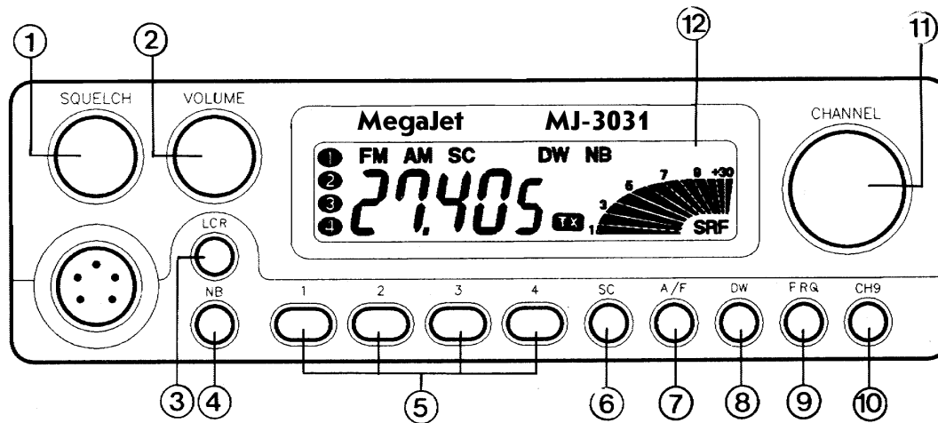
Рис.1. Радиостанция MegaJet MJ-3031. Вид панели управления.
