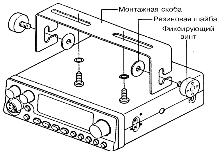
Рис.2. Крепление радиостанции при помощи монтажной скобы.
